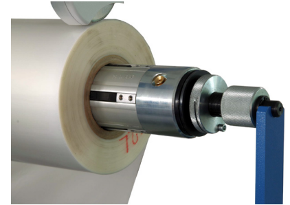
Optional Air shaft
